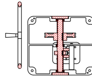
断面図 B-B
